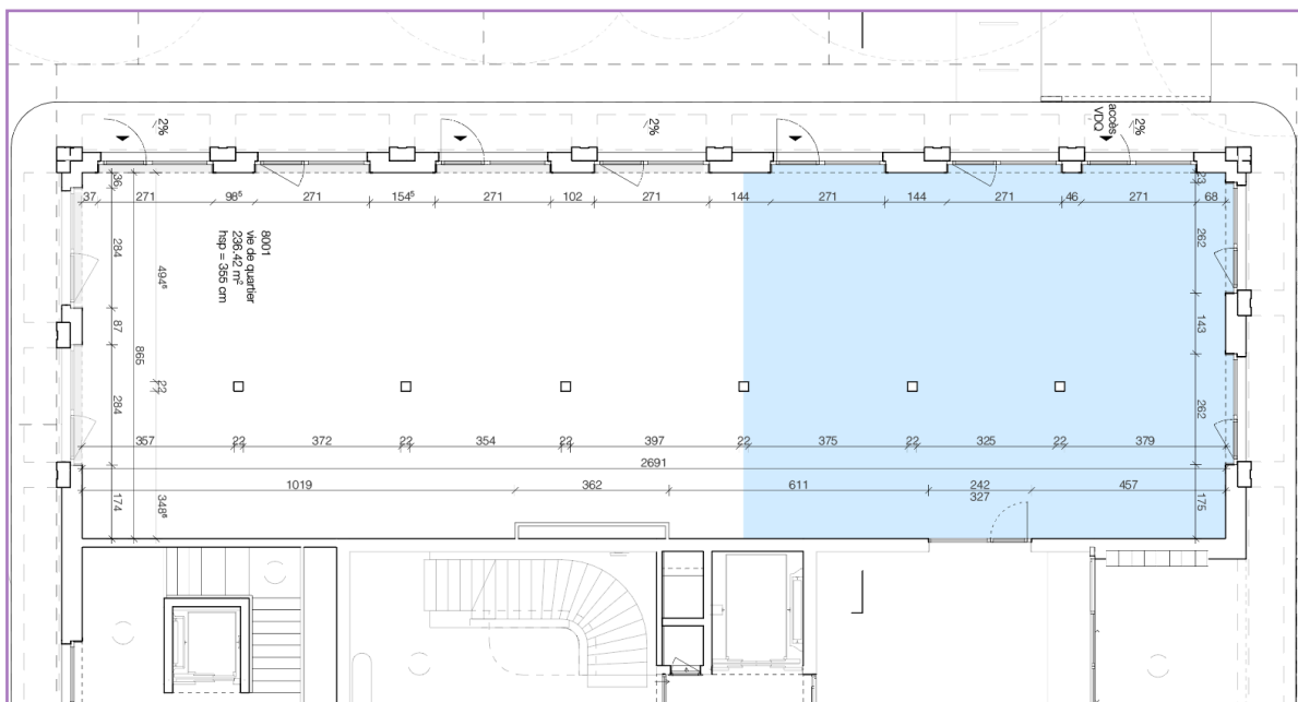
Plan de l'arcade (uniquement la zone correspondant à l'aplat bleu)
